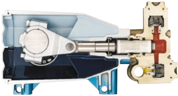
CP Pumps
